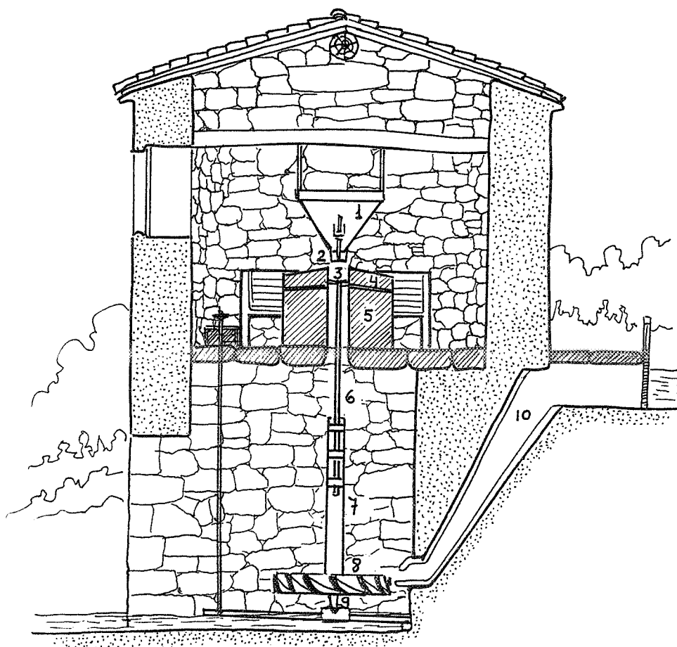
Esquema dun muíño de rodicio
